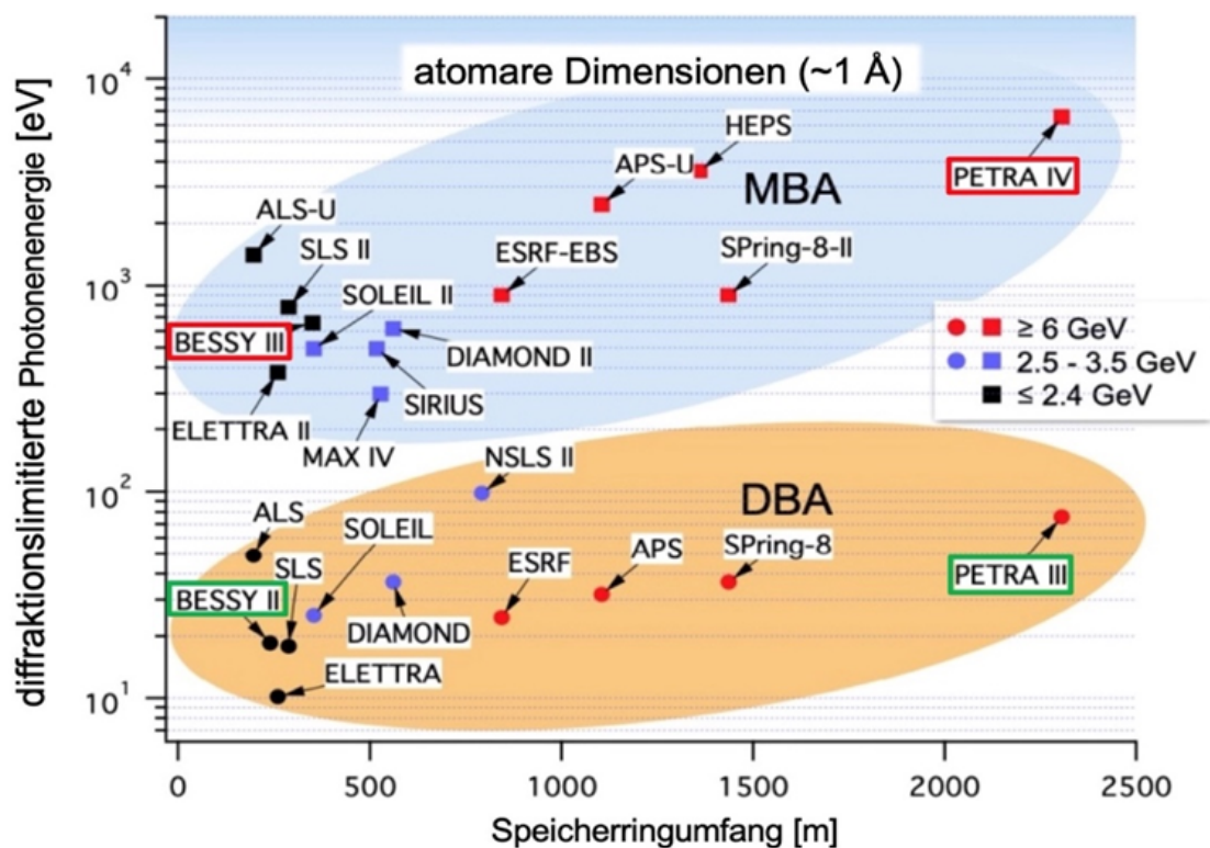
Abbildung 6.1: Darstellung der Photonenergie, bis zu der eine Quelle beugungsbegrenzt ist, d.h. bis zu der Photonenergie die theoretisch mögliche Brillanz erreicht wird, als Funktion des Umfangs. DBA: Double-Bend-Achromat, Quellen der 3. Generation; MBA: Multi-Bend-Achromat, Quellen der 4. Generation. DALI ist hier, da kein Speicherring, nicht aufgeführt (ein internationaler Vergleich ist in Tabelle 6.3 zu finden).
