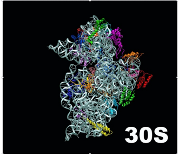
Abbildung 2.2: Links: Ada Yonath beim Experimentieren an einer Synchrotronstrahlungsquelle. Rechts: Schematische Struktur der 30S-Untereinheit des Ribosoms.
